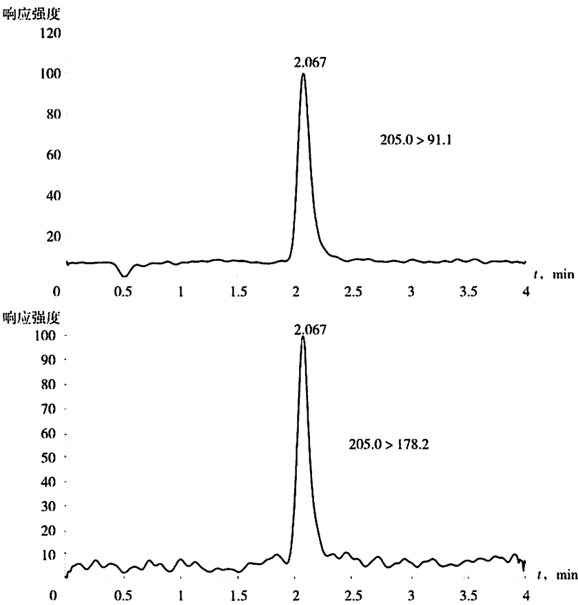
图 A. 1 左旋咪唑标准溶液特征离子质量色谱图(2. 5 µg/L)
