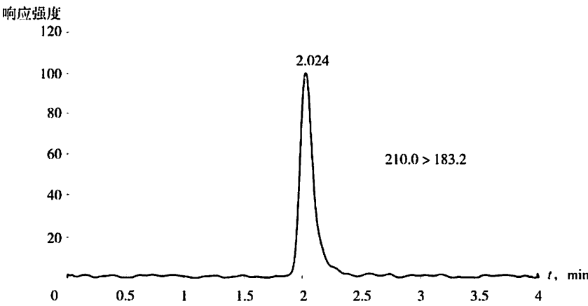
图 A. 2 左旋咪唑-D 5 标准溶液的特征离子质量色谱图(10 µg/L)
