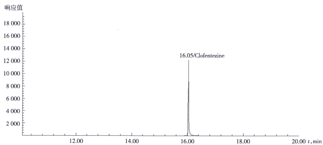
图 B. 1 四螨嗪标准品的气相色谱—质谱选择离子色谱图
