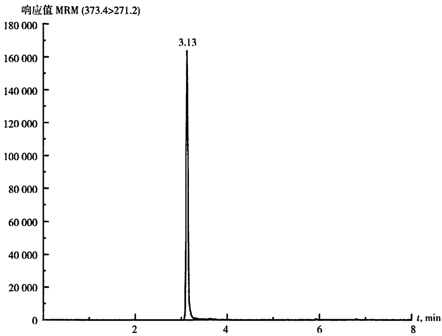
图 B.6 醋酸羟孕酮(HPA)标准溶液定量离子色谱图( RT=3.13\text{ min} )
