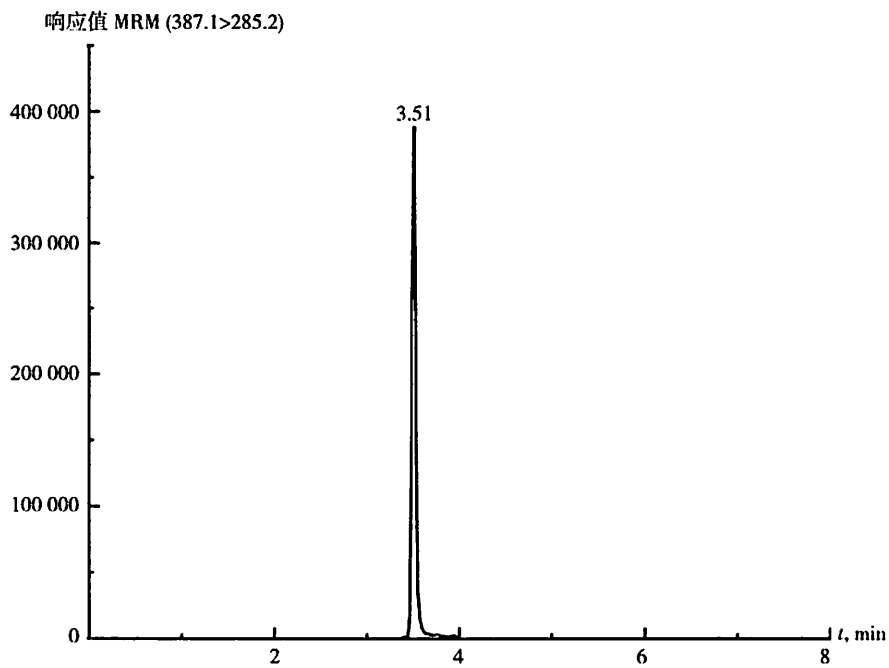
图 B.5 醋酸甲羟孕酮(MPA)标准溶液定量离子色谱图( RT=3.51\text{ min} )
