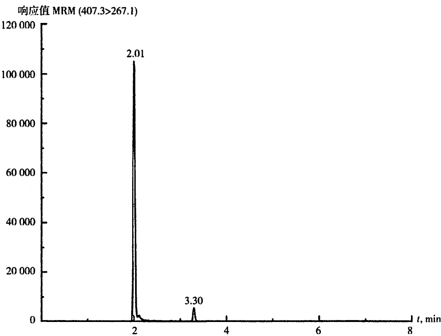
图 B.1 醋酸氟孕酮(FGA)标准溶液定量离子色谱图( RT=2.01 min)
