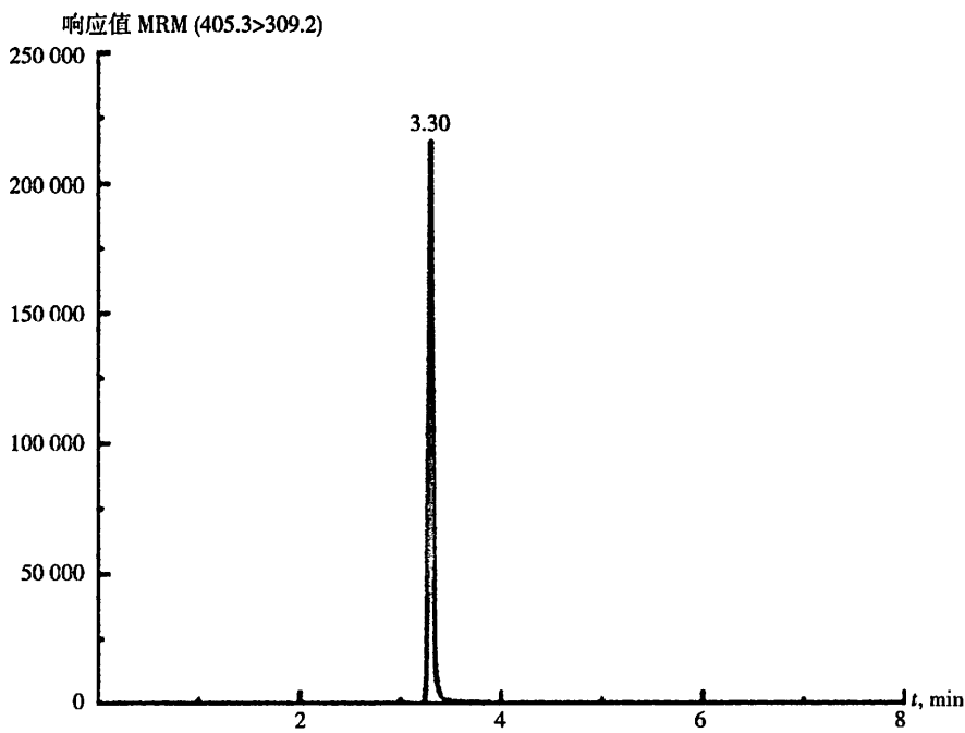
图 B.4 醋酸氯地孕酮(CMA)标准溶液定量离子色谱图( RT=3.30 min)
