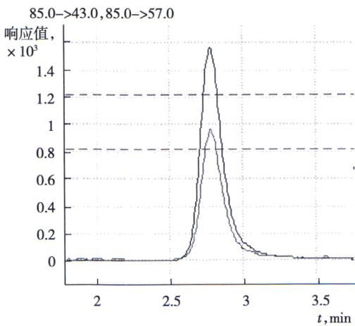
图 B.2 表 1 中条件 2 下杀草强液相色谱—质谱/质谱多反应监测色谱图
