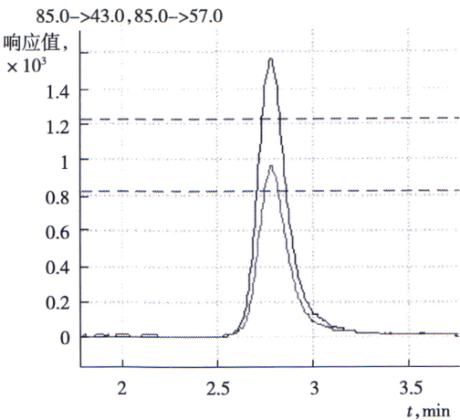
图 B.1 表 1 中条件 1 下杀草强液相色谱—质谱/质谱多反应监测色谱图
