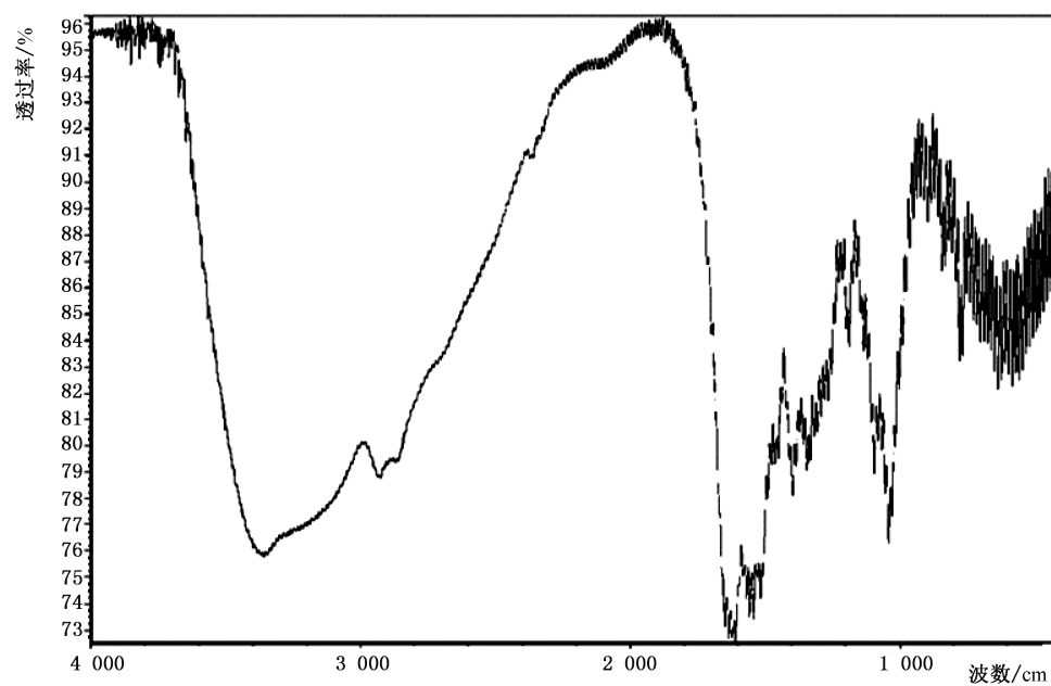
图 B.1 (6S)-5-甲基四氢叶酸,氨基葡萄糖盐参考红外光谱图
