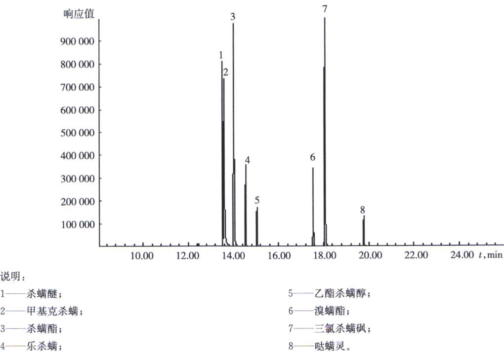
图 C.1 8 种杀螨剂标准物质总离子流图
