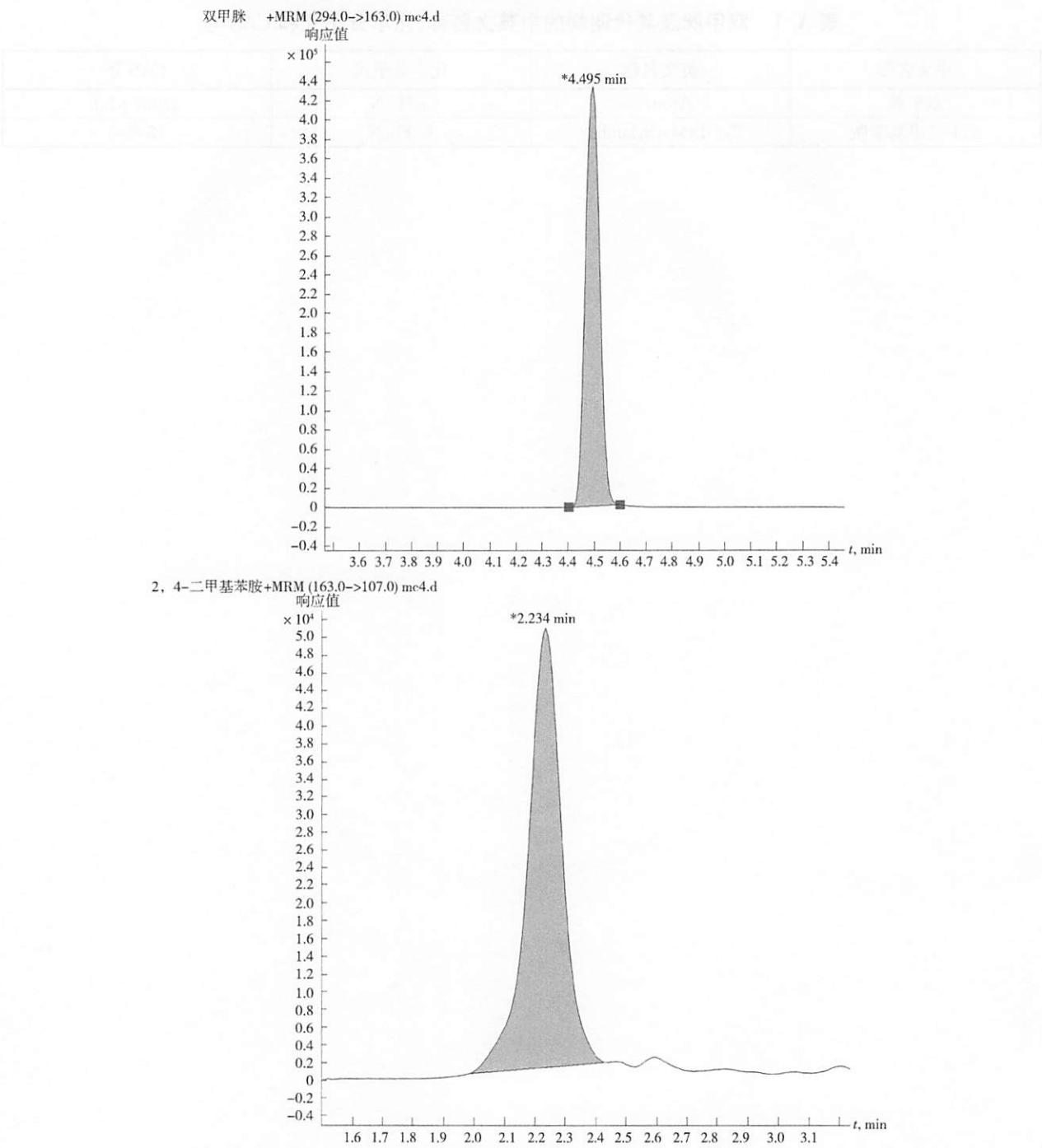
图 B.1 双甲脒及其代谢物 2,4-二甲基苯胺混合标准溶液的特征离子质量色谱图(2.5 ng/mL)
