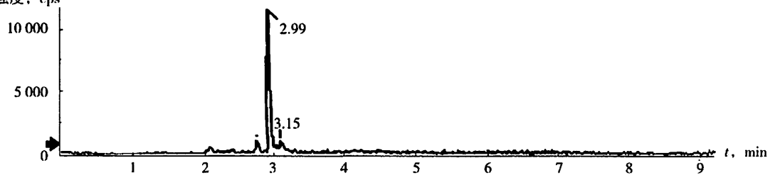
图 A.1 去吠喃甲酰基头孢噻呋标准溶液特征离子质量色谱图(4 μg/L)
