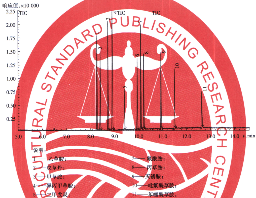
图 C.1 11 种除草剂标准物质气相色谱—质谱选择离子色谱图
