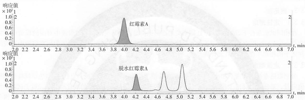
图 A. 1 红霉素 A 及其降解物混合标准溶液(10 \mu\text{g/L} )的定量离子色谱图
