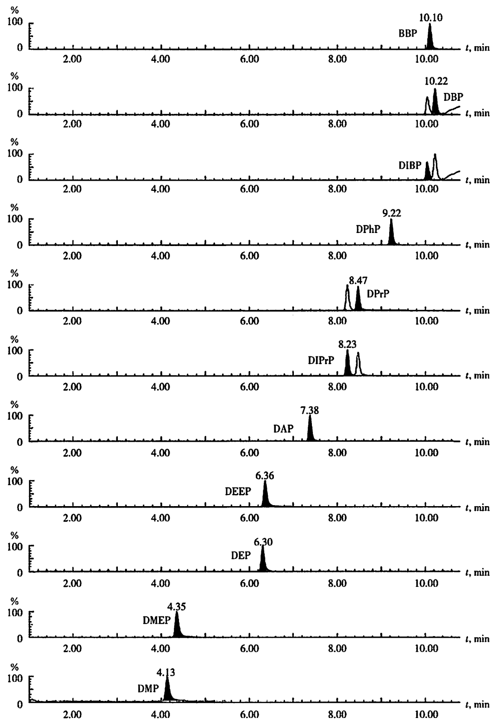
图 B. 1 邻苯二甲酸酯类物质标准工作液的定量特征离子质量色谱图(10 ng/mL)
