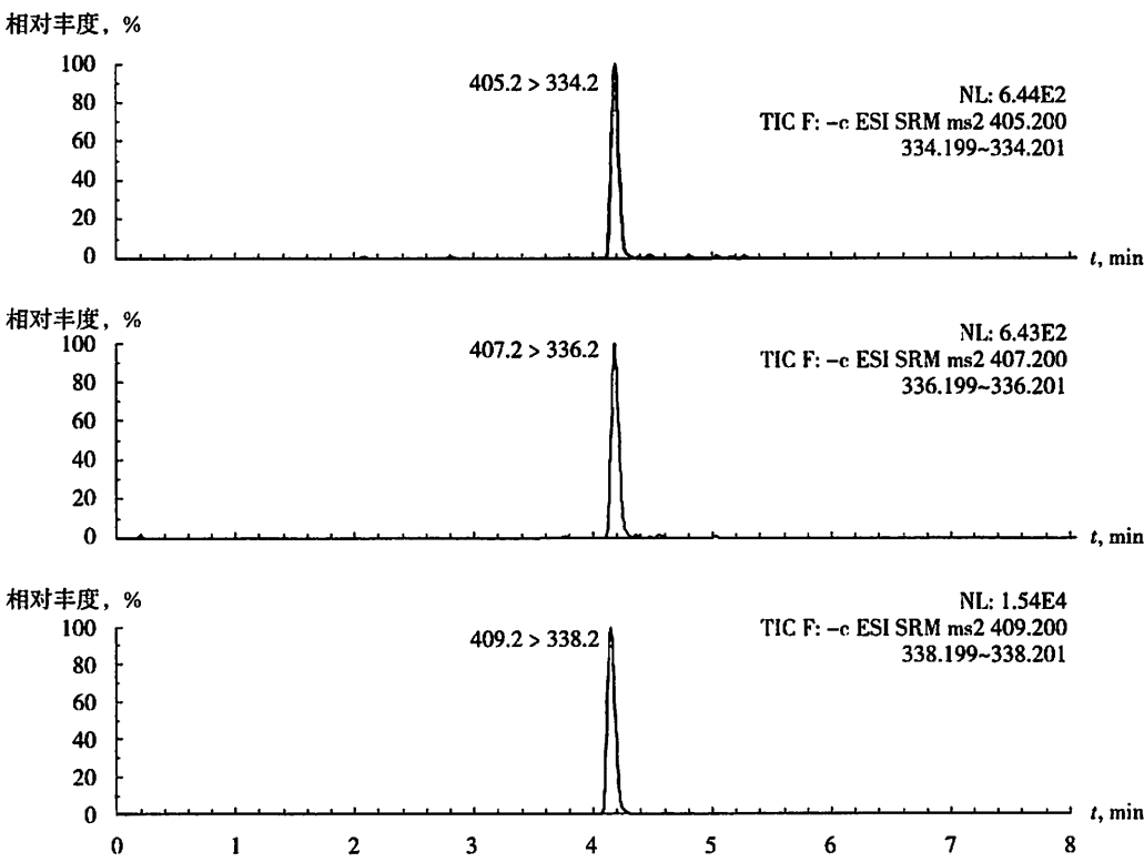
图 A. 1 地克珠利和地克珠利- d_4 标准溶液特征离子质量色谱图(2 ng/mL)
