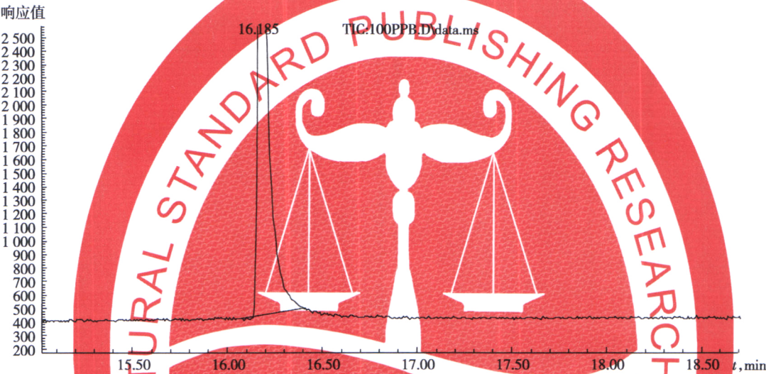
图 A.1 吡螨胺标准物质总离子流色谱图
