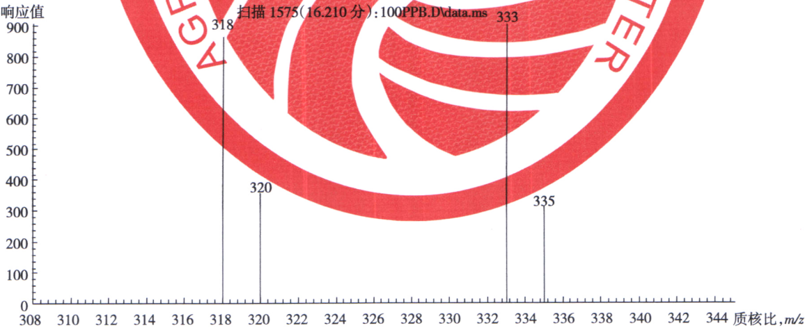
图 A.2 吡螨胺标准物质的质谱图
