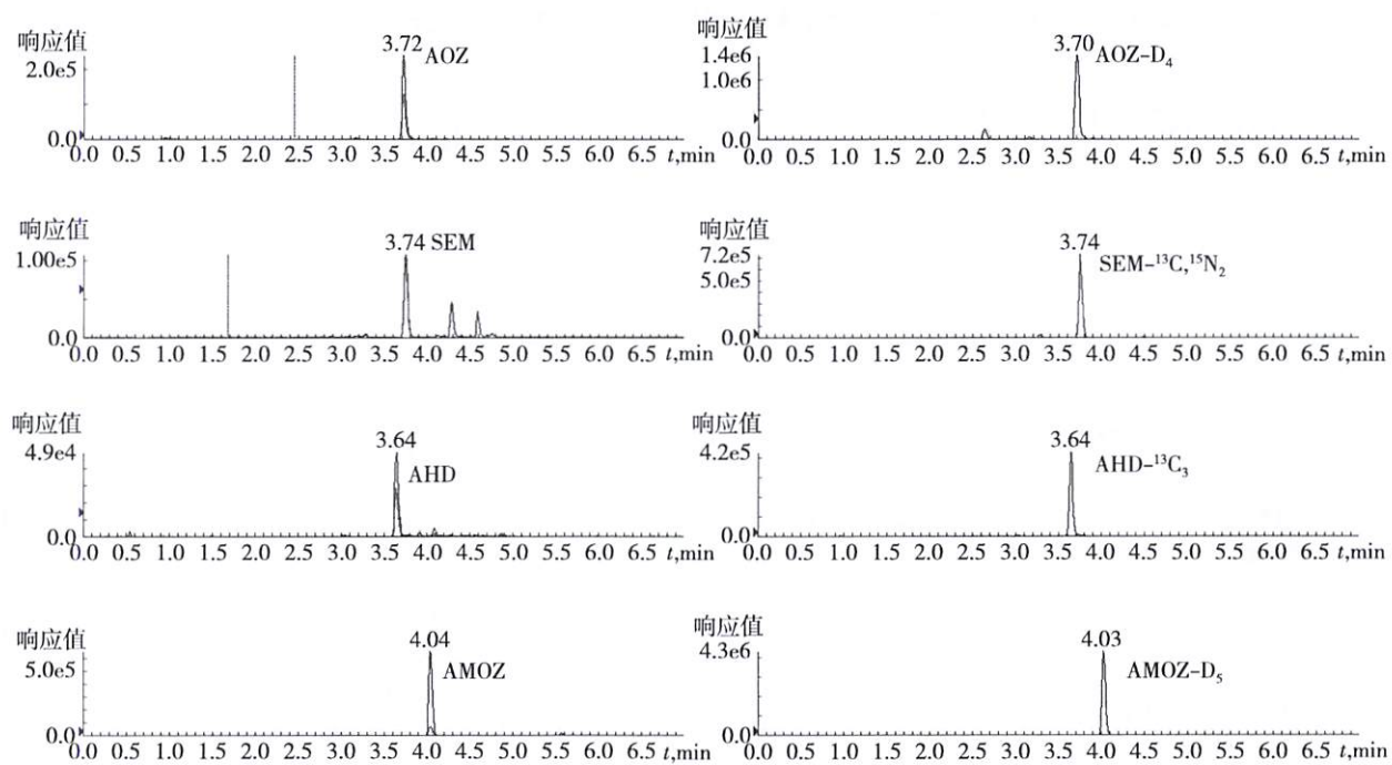
图 B.1 硝基呋喃类代谢物标准溶液特征离子质量色谱图(2.0 μg/L)
