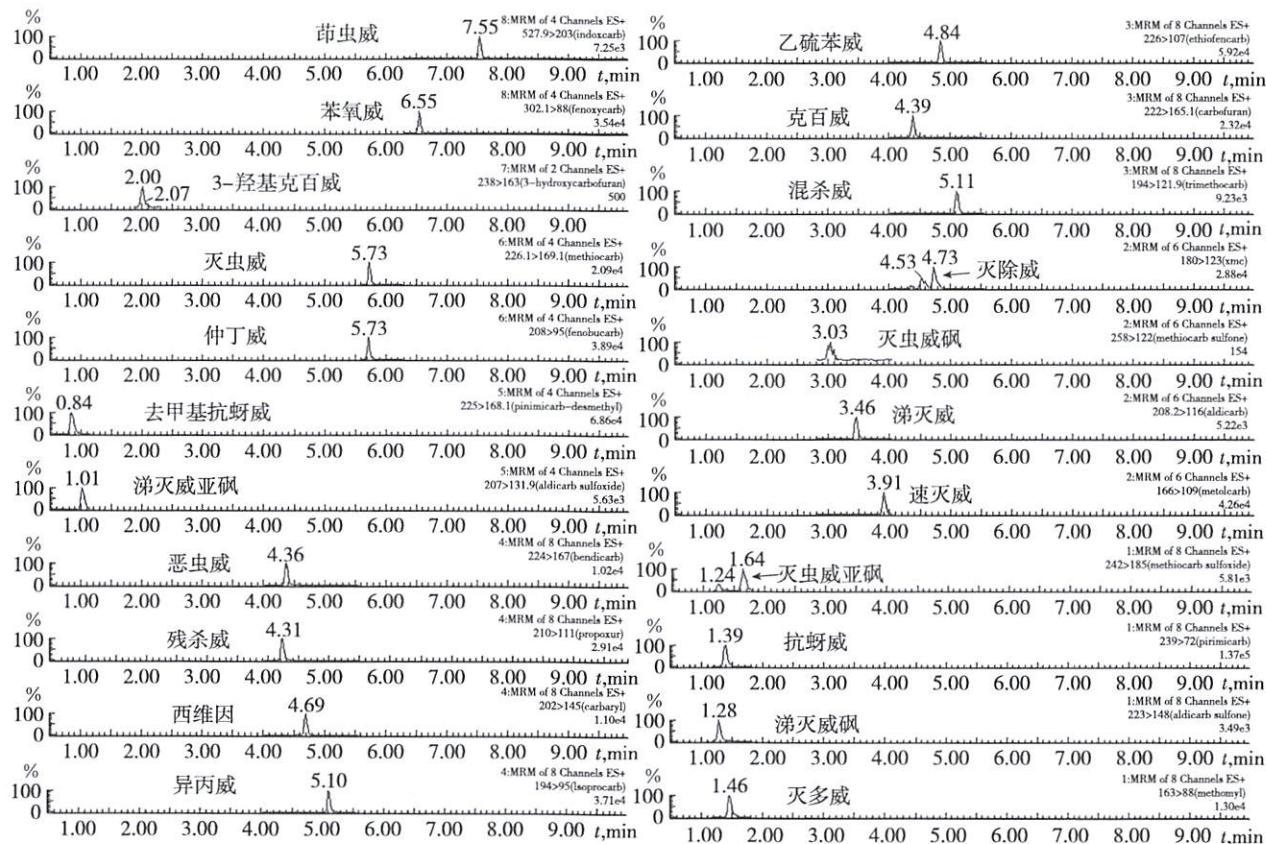
图 B.1 氨基甲酸酯类杀虫剂标准溶液(5.0 µg/L)MRM 色谱图
