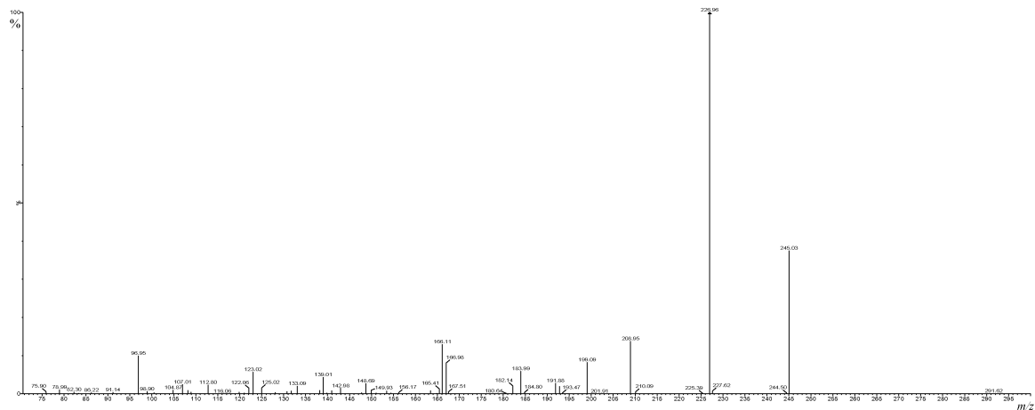
图 A.1 生物素标准溶液(100 \mu\text{g/L} )质谱扫描图
