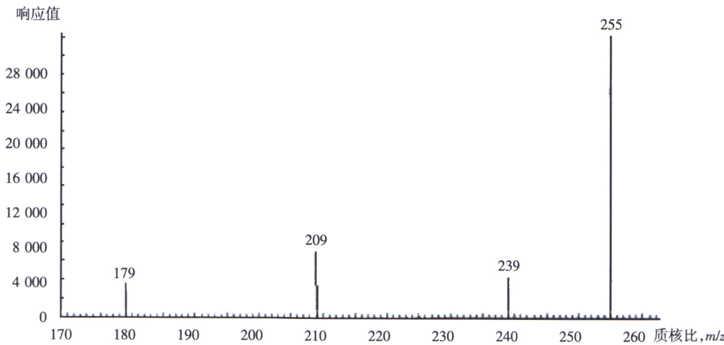
图 A.2 4,6-二硝基邻甲酚-MTBSTFA 衍生物 SIM 质谱图
