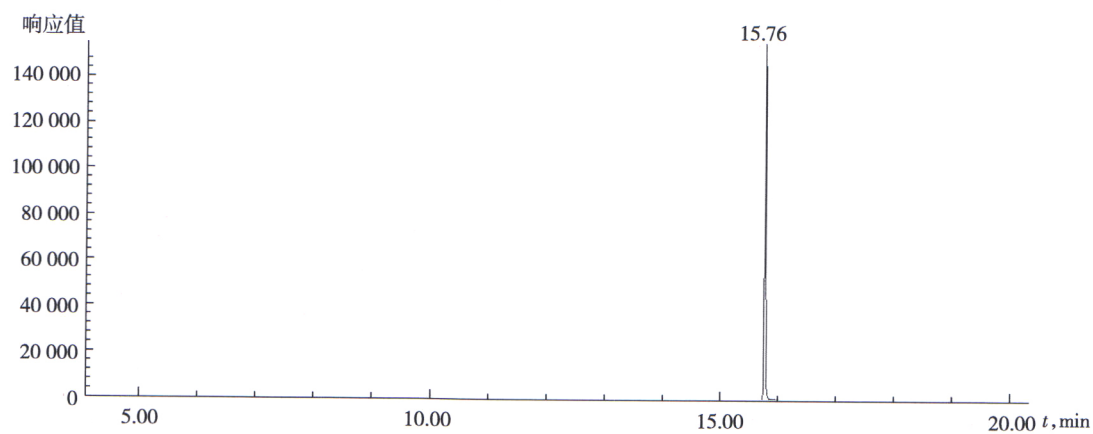
图 B.1 野燕枯标准物质的气相色谱—质谱选择离子色谱图
