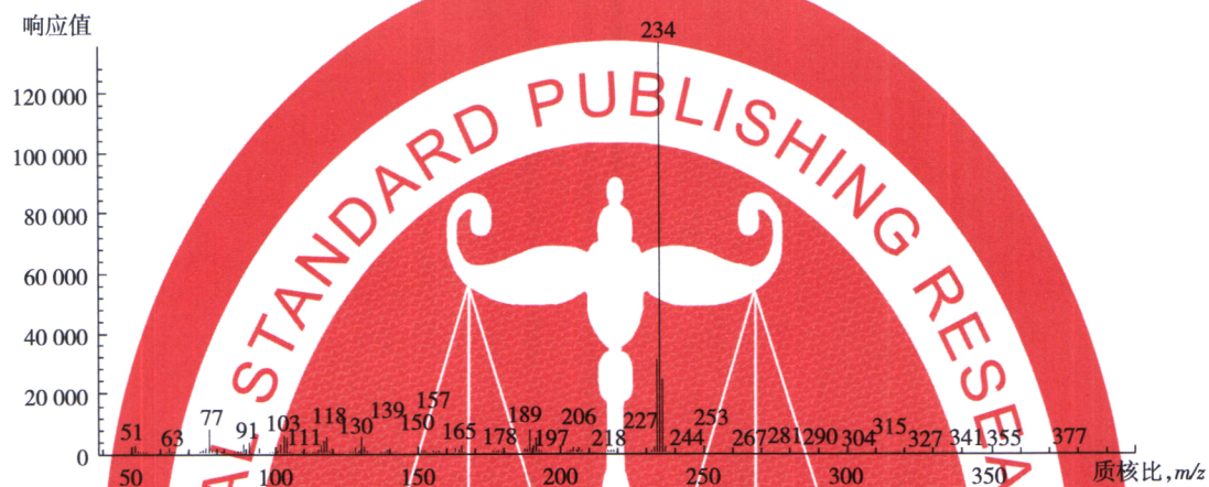
图 C.1 野燕枯标准品的气相色谱—质谱图
