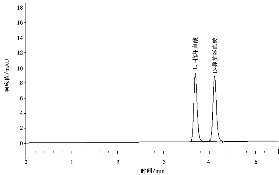
图 A.1 L-抗坏血酸(1.0 \mu\text{g/mL} )、D-异抗坏血酸(1.0 \mu\text{g/mL} )标准溶液色谱图
